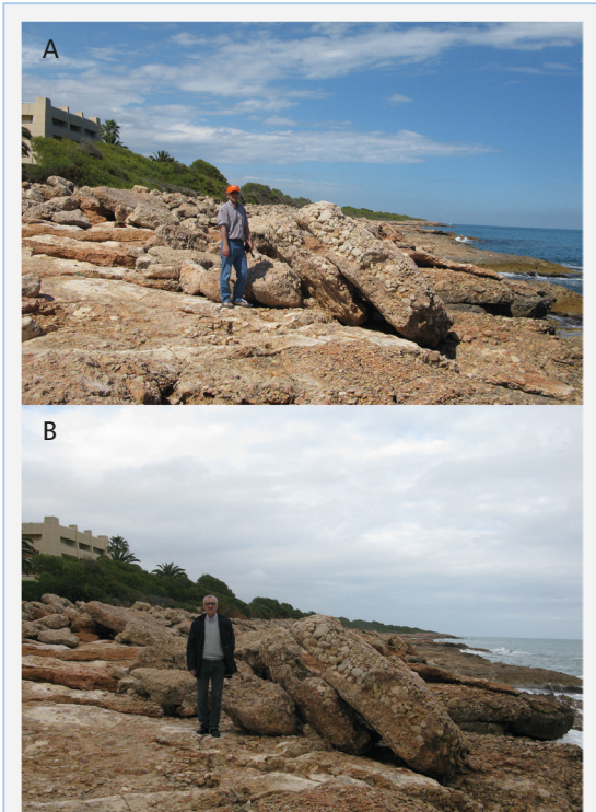
FIGURA 3. Blocs de tsunami al pla de Roda (serra d'Irta), comparança temporal. A: foto del 31/05/2018 (Roig-Munar et al., 2018b: 17; Fig. 4A. B: foto del 18/02/2020, després de la tempesta Glòria.
